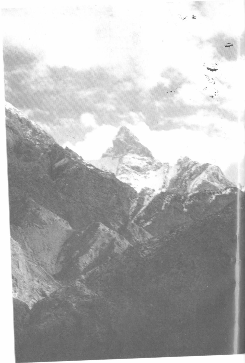
Помири Ғарбӣ. Пирях дар доманаи қаторкӯҳи Академияи илм
