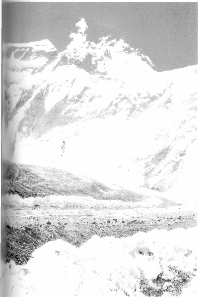
Пиряхи кӯҳсори Зарафшон.
