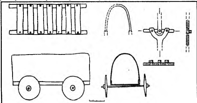
Расми 46 а. Сохти аробаи нӯшишдор.
