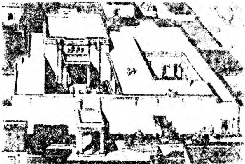
Расми 70. Намуди барқароркардаи маъбади Гад аз Дураевронос.
