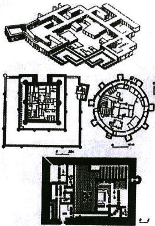
Расми 24. Меъмории Бохтар ва Маргиён. 1) Кохи шохи Даштӣ-3, 2) Маъбади Тоголок-21. 3) Маъбади Даштӣ-3, 4) Маъбади Чаркӯтан.
