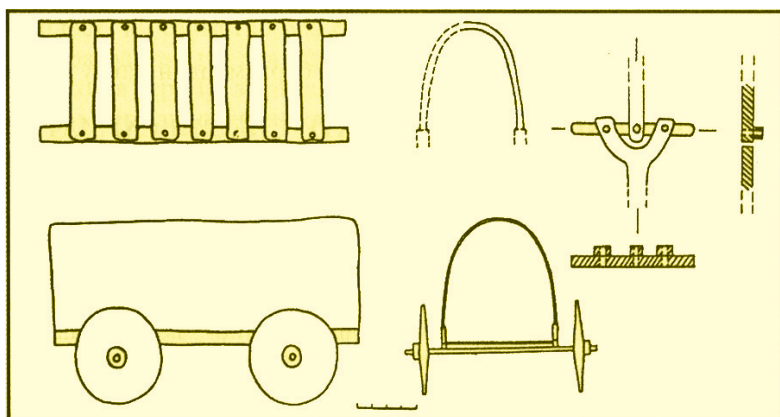
Расми 46 а. Сохти аробаи нӯшишидор.
