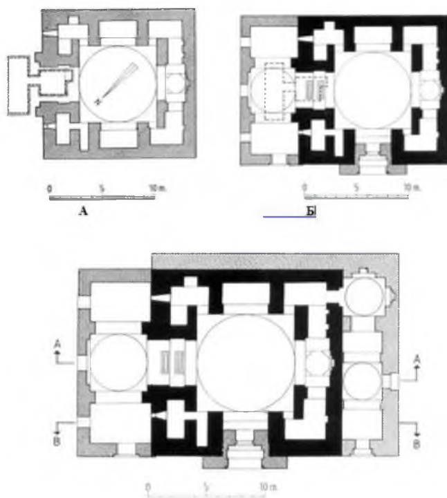
Илл. 7. Мавзолей Мухаммада Башоро. Реконструкция плана: А - 1-ого строительного периода; Б - 2-ого строительного периода; В - 3-ого строительного периода (Хмельницкий, 2013).
