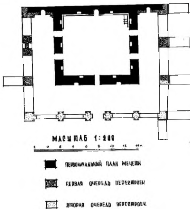
Илл. 5. Общий план Медресе – мечети Олима Додхо в Пенджикенте (Каримова, 2016).
