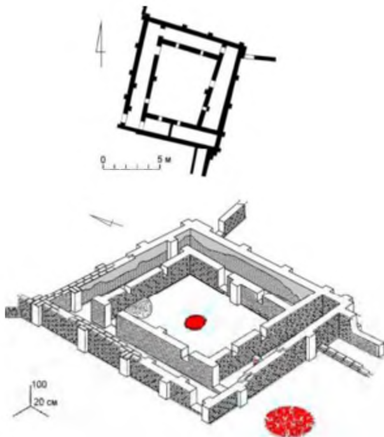
Илл. 1. Саразм. Храм огня, Раскоп XI, горизонт 2, план и аксонометрия (Раззоков, Худжагелдиев, 2010).
