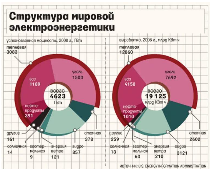
Расми 2. Сохтори электроэнергетикаи ҷаҳон дар соли 2008: а) иқтидорҳо бо ГВт, б) истеҳсоли энергия бо млрд кВт·соат 6
