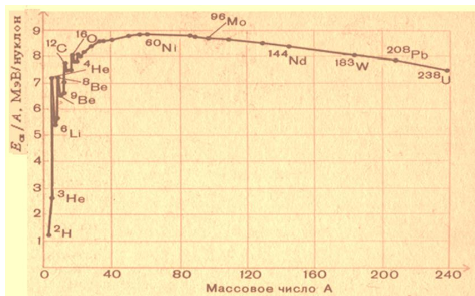
Расми 1. Вобастагии энергияи бандиши хос аз адади массавии ядро
